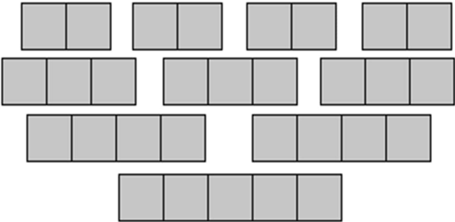
Schiffe Spieler 1
