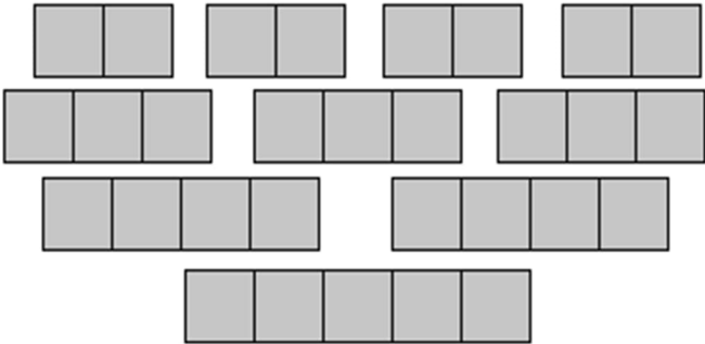
Schiffe Spieler 2
